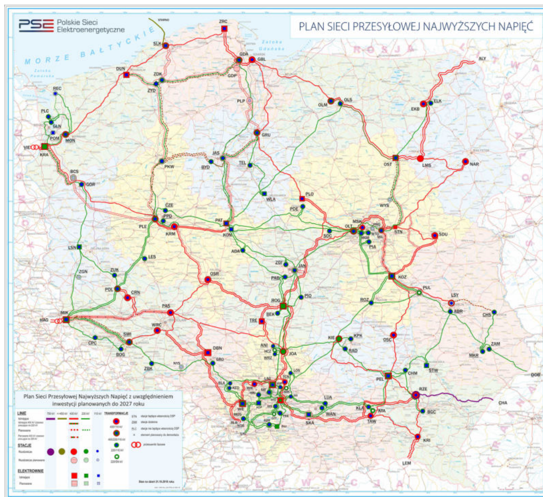
Plan Sieci Przesyłowej Najwyższych Napięć
